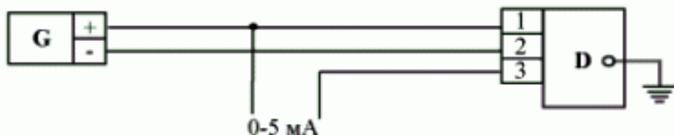
в) Датчик с выходным сигналом 0 - 5 мА, 3-проводная линия
