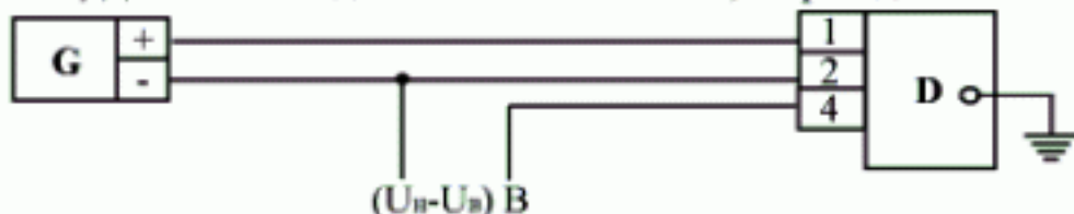
г) Датчик с выходным сигналом (U_n - U_B) В, 3-проводная линия
